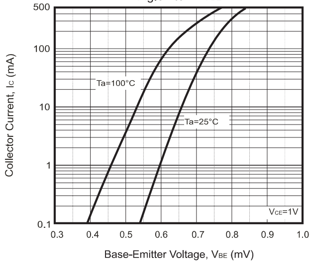
Fig.5 - I_C - V_{BE}
